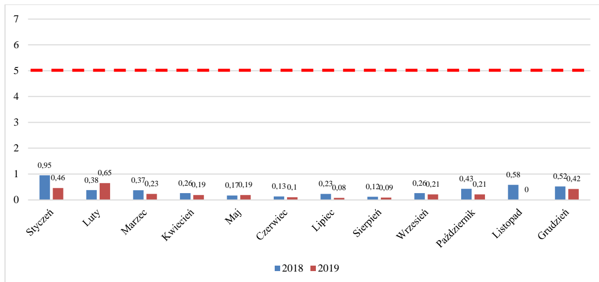
Rysunek 14 Wyniki pomiarów stężenia kadmu - stacja w Zgorzelcu - \mu\text{g}/\text{m}^3
