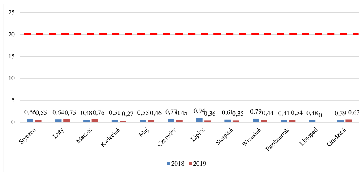
Rysunek 15 Wyniki pomiarów stężenia niklu - stacja w Zgorzelcu - \mu\text{g}/\text{m}^3
